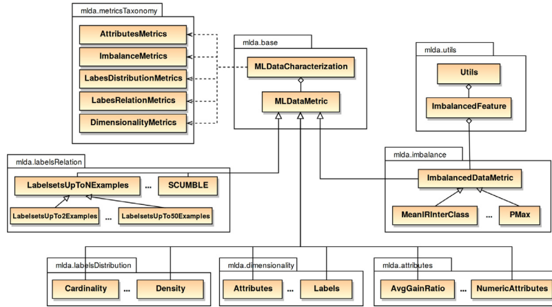
Fig. 1. MLDA class diagram.
